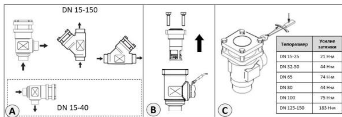
Рис. 3 – Монтаж клапана
