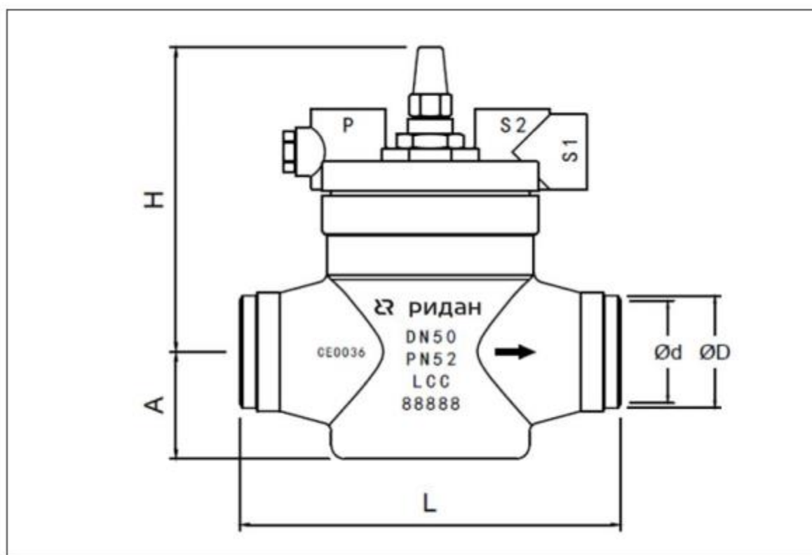
Рисунок 2. Размеры
