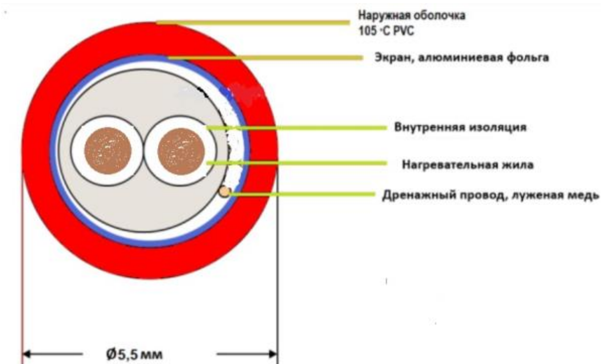
Рис. 2.2. Устройство нагревательного кабеля ДЕВИ Flex-18T. Поперечный разрез.
