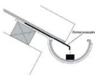
Датчик в желобе (дополнительный козырек)
