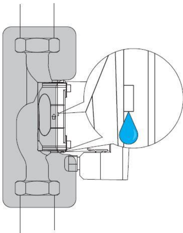
Рис. 8. Теплоизоляция насоса
