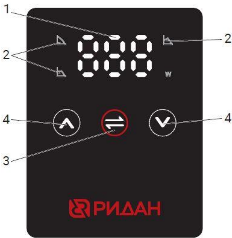
Рис. 4. Панель управления насосом RWE 32-120S.
