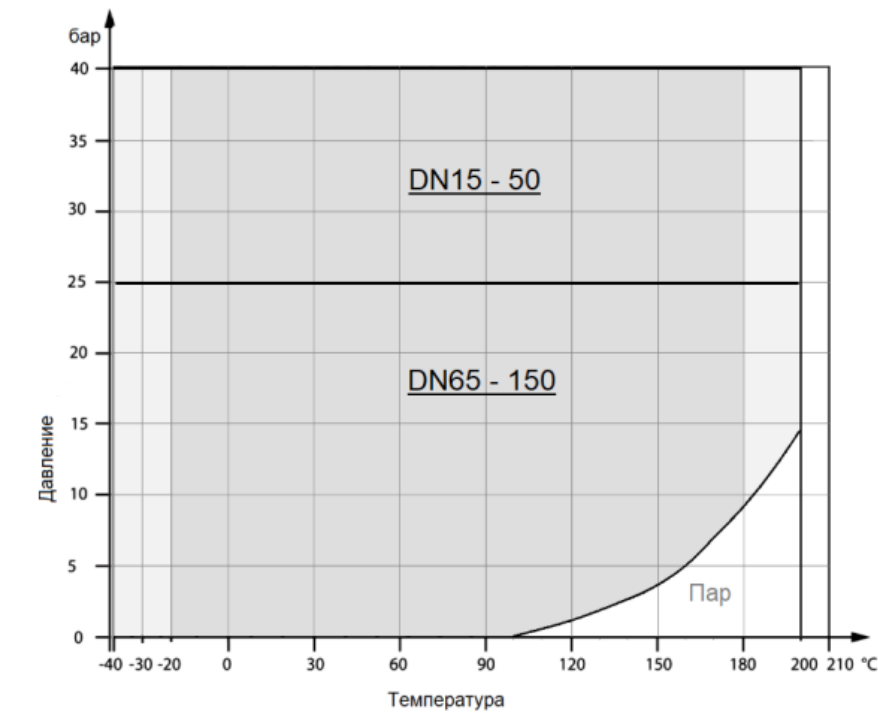
График Температура-Давление
