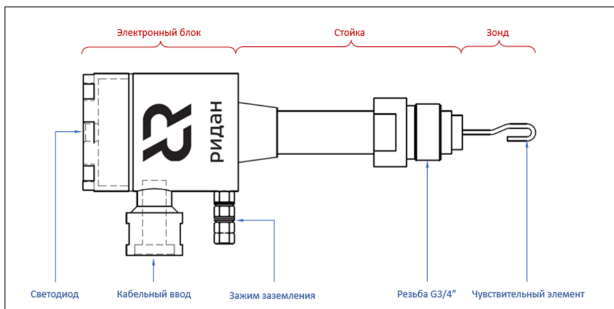
Рис. 3 – Конструкция
