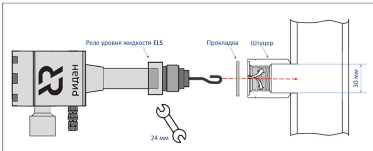
Рис. 4 – Монтаж
