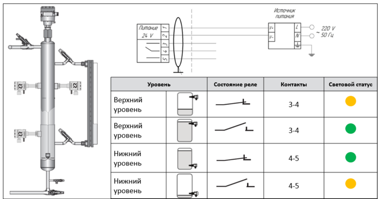
Рис. 5 – Электрическое подключение
