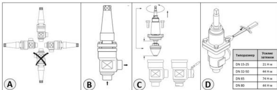
Рис. 3 – Монтаж клапана
