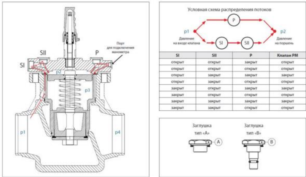
Рисунок 3. Принцип работы
