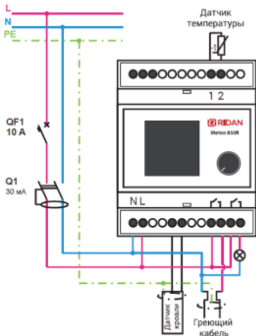
Схема подключения терморегулятора Ридан Meteo 850R при максимальном токе нагрузки греющего кабеля меньше 10 А
