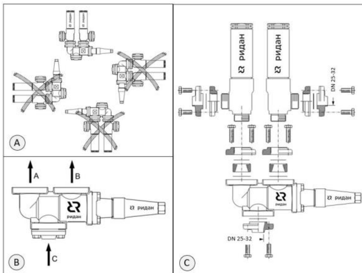
Рис. 3 - Монтаж
