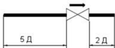
рис.3: Правила монтажа
