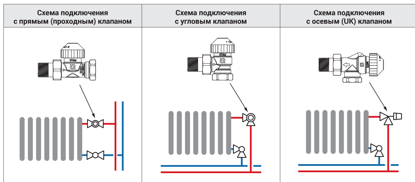
Рис.7 Схема подключения отопительных приборов
