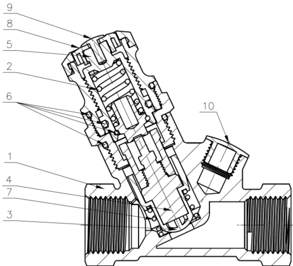
1 — корпус; 2 — пружина безопасности; 3 — золотник; 4 — термоэлемент; 5 — настроечная рукоятка; 6 — кольцевые уплотнения; 7 — пружина; 8 — шкала настройки; 9 — заглушка отверстия для ключа; 10 — отверстие для термометра Рис. 2 - Устройство клапана АНТ-R
