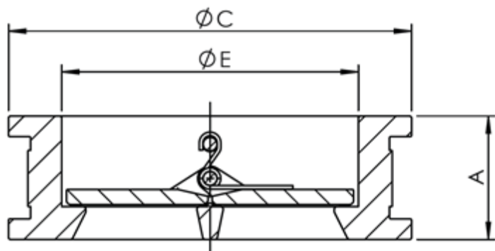
Габаритные и присоединительные размеры затворов обратных тип NVD-895R
