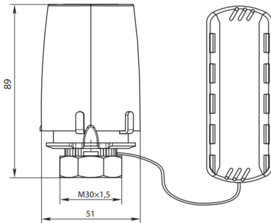
Рис. Габаритные размеры термоэлемента
