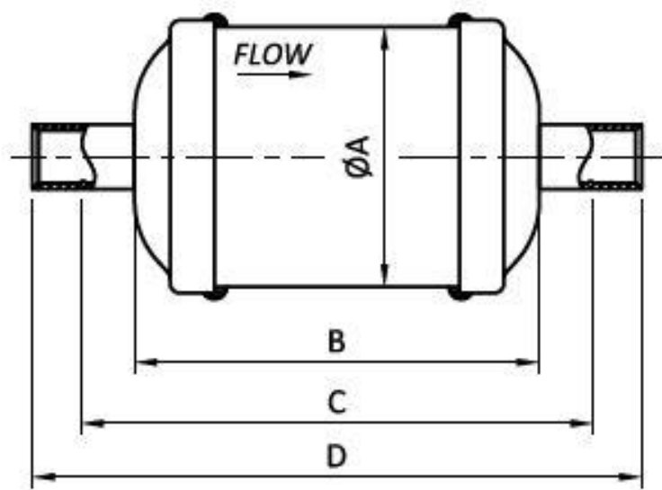
Типоразмер DFL 05-75
