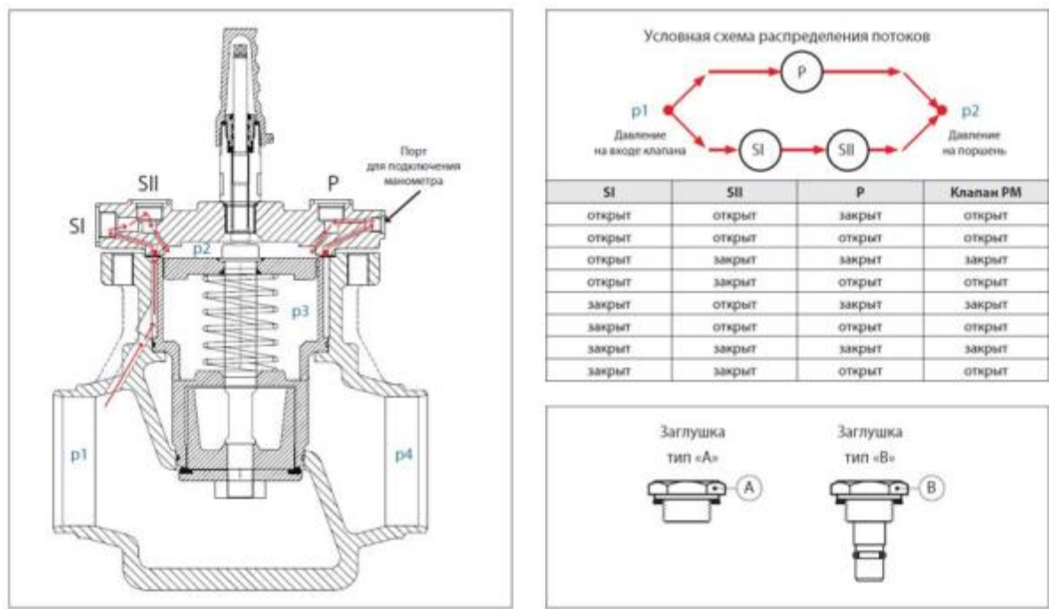
Рисунок 3. Принцип работы
