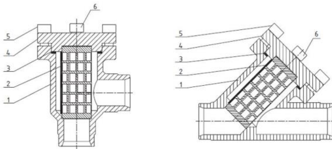
Рис. 1 – Конструкция
