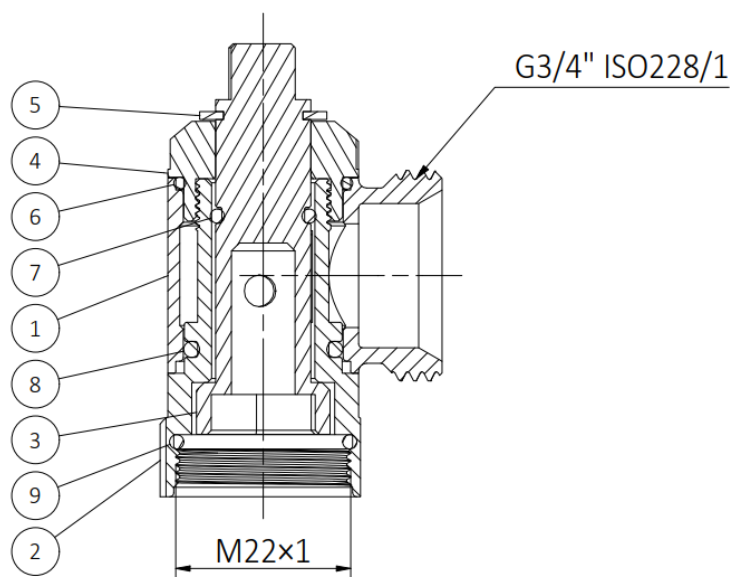
Дренажное устройство 003L0152R: 1) Поворотный корпус; 2) Гайка крепления к клапану; 3) Ключ; 4) Гайка; 5) Стопорное кольцо; 6), 7), 8), 9) Кольцевые уплотнения.
