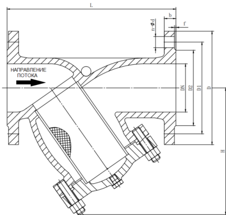
Габаритные размеры фильтров сетчатых типа ФСФ
