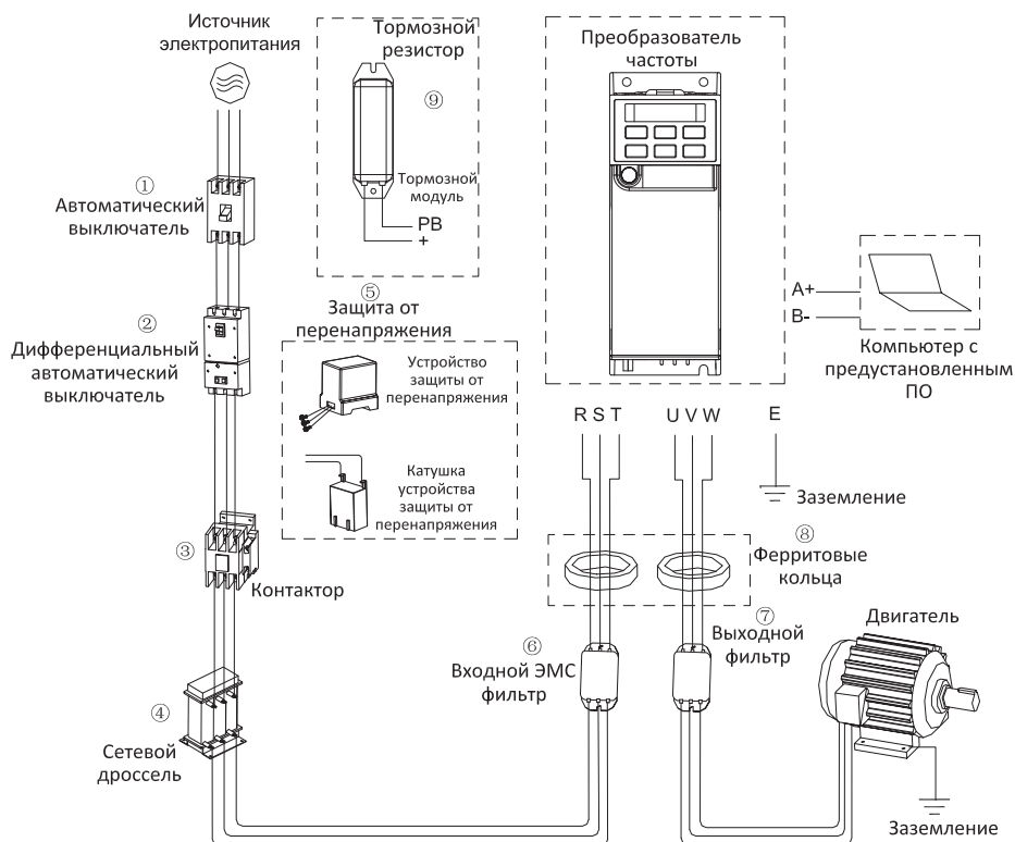
Рисунок 6.3-1 – Подключение внешних устройств
