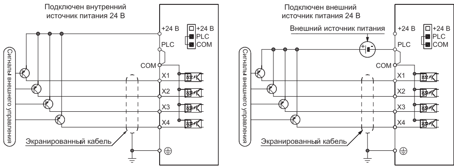
Рисунок 4.7-1 – Способ подключения логики PNP для мощностей 7,5–22 кВт
