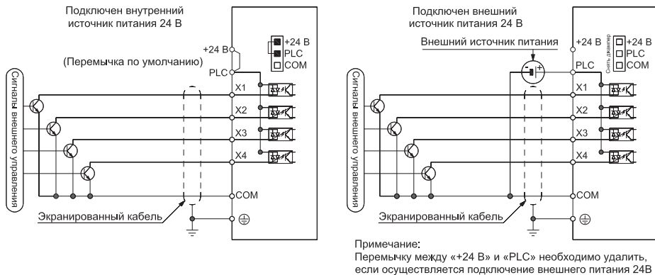
Рисунок 4.7-2 – Способ подключения логики NPN (перемычку между «+24 В» и «PLC» необходимо удалить, если осуществляется подключение внешнего питания 24 В) для мощностей 7,5–22 кВт
