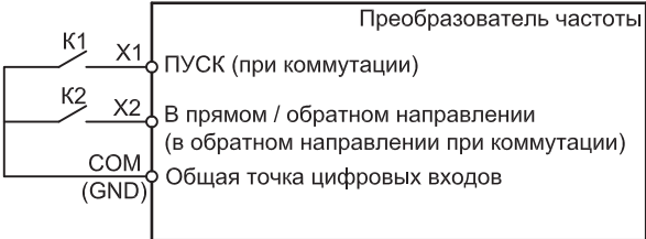
Рисунок 10.9-6 – Двухпроводная схема управления 2
