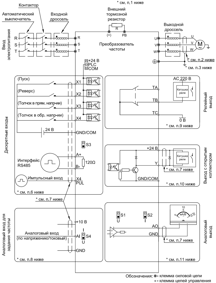
Рисунок 4.5-2 – Схема внешних подключений для PNP-схемы подключения цифровых входов
