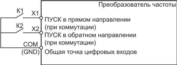
Рисунок 10.9-5 – Двухпроводная схема управления 1
