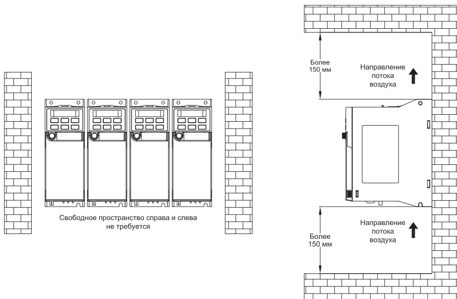
Рисунок 3.5-1 – Положение преобразователя частоты и требуемое пространство.
