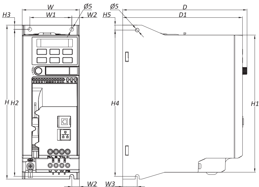
Рисунок 3.6-4 – Чертеж преобразователя частоты типоразмера А2 без защитной крышки
