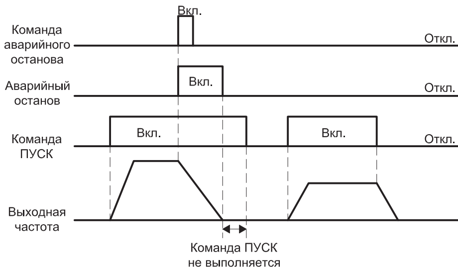
Рисунок 10.9-1 – График, совмещающий команды ПУСК и аварийный останов
