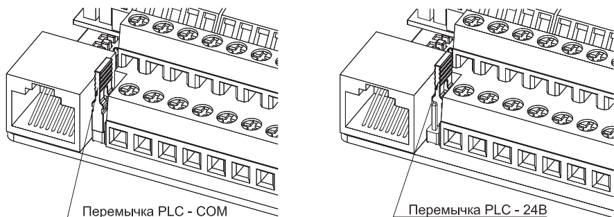
Рисунок 4.7-3. Схема подключения перемычек «+24 В», «PLC», «COM» для мощностей 7,5–22 кВт
