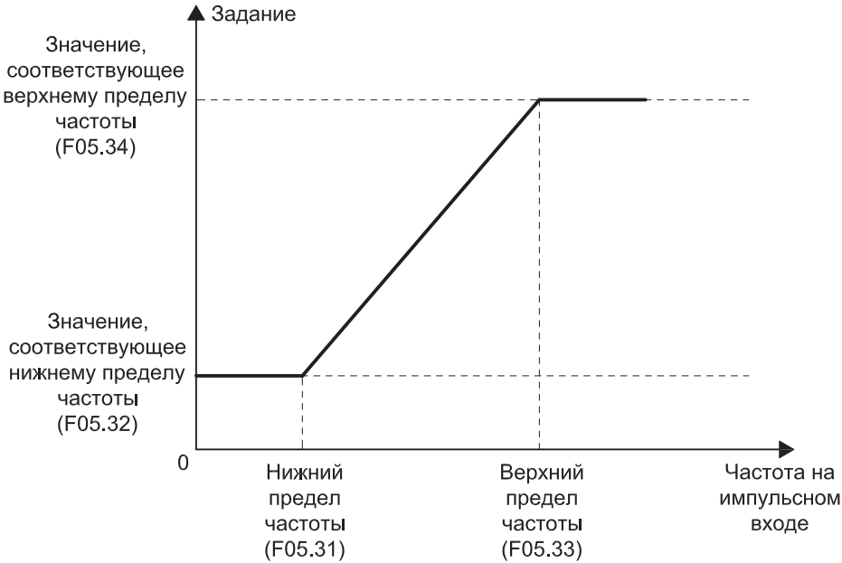
Рисунок 10.9-9 – Обработка частоты сигнала, поступающего на импульсный вход
