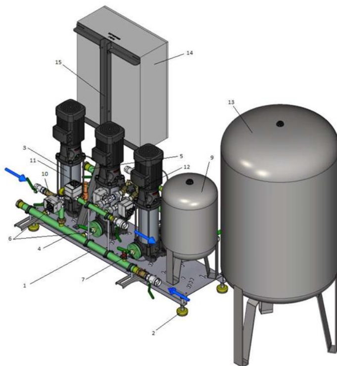
Рисунок 4 - Внешний вид установки насосной тип WaterJump-FS
