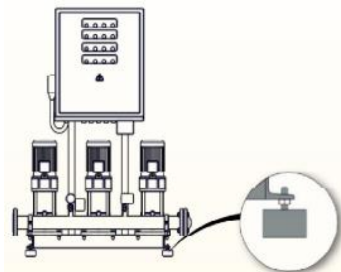
Рисунок 14 - Регулируемые виброопоры
