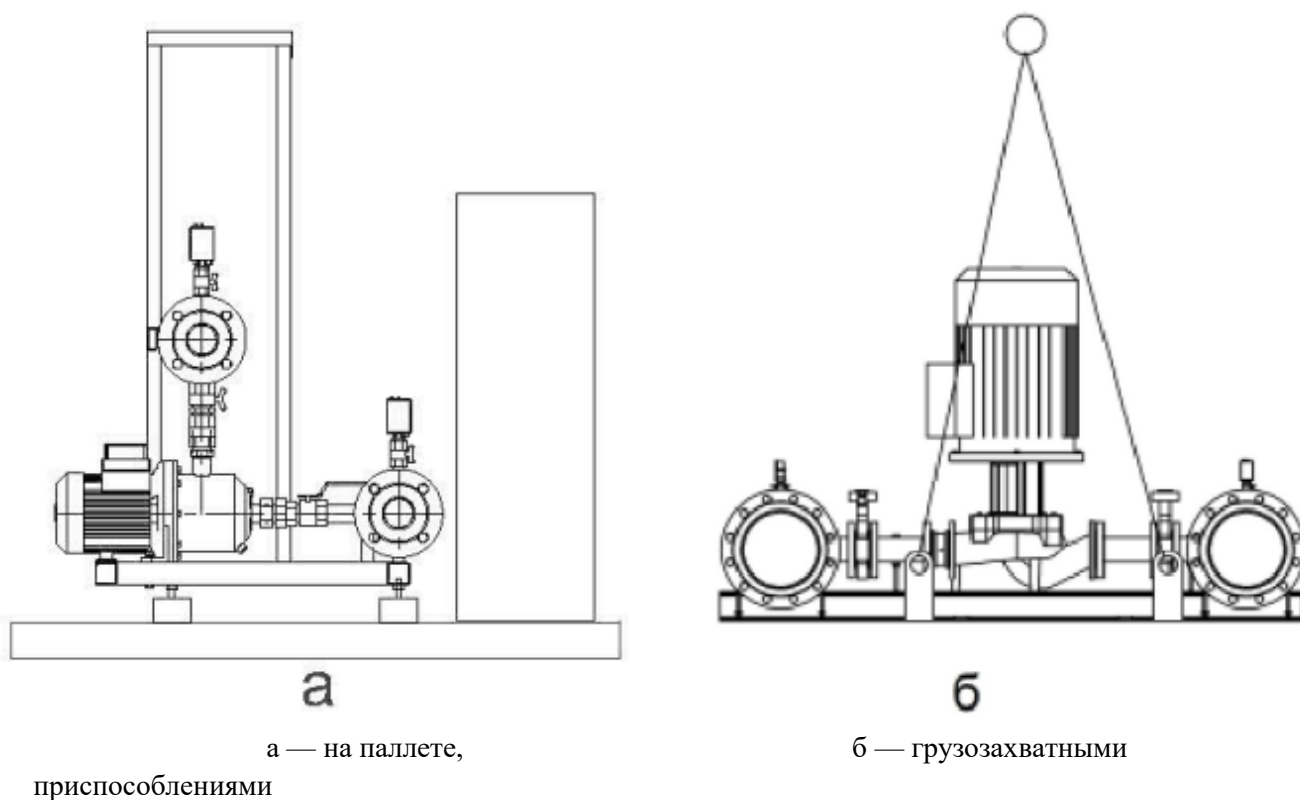
Рисунок 16 — Подъем/захват установок
