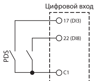
Пример схемы подключения на цифровые входы, сухой контакт
