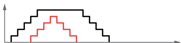
Время/LIFO CCpp
