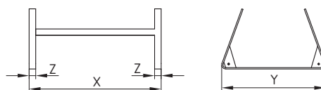
Опорная рама для DN300–600
