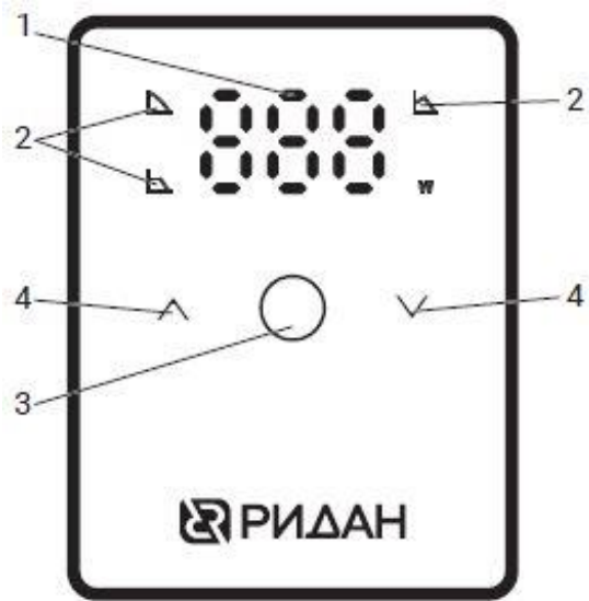
Рис. 4. Панель управления насосом RWE 32-120S.
