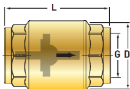
Габаритные и присоединительные размеры клапана обратного
