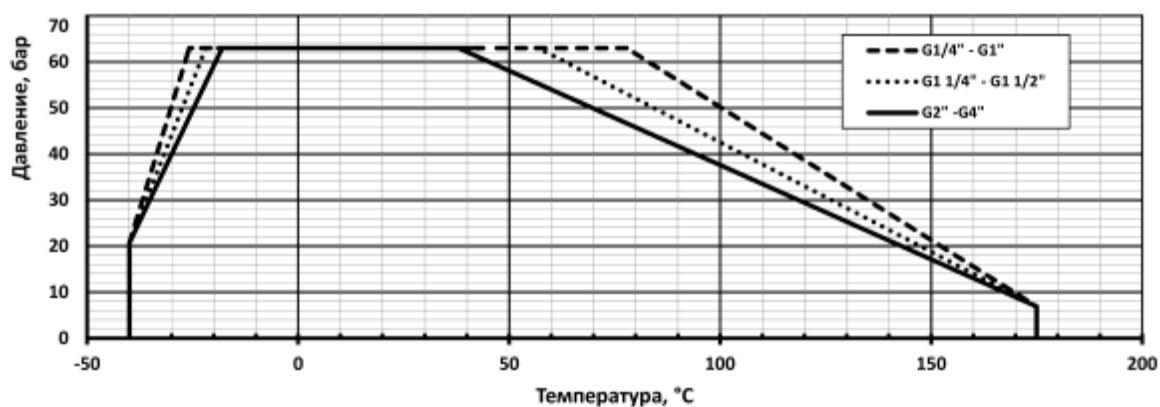
Температура-Давление
