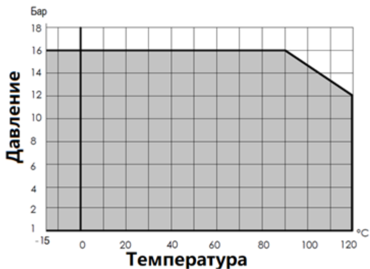
Диаграмма Температура-Давление
