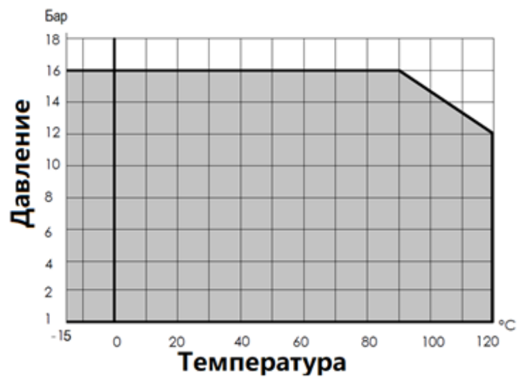
Диаграмма Температура-Давление
