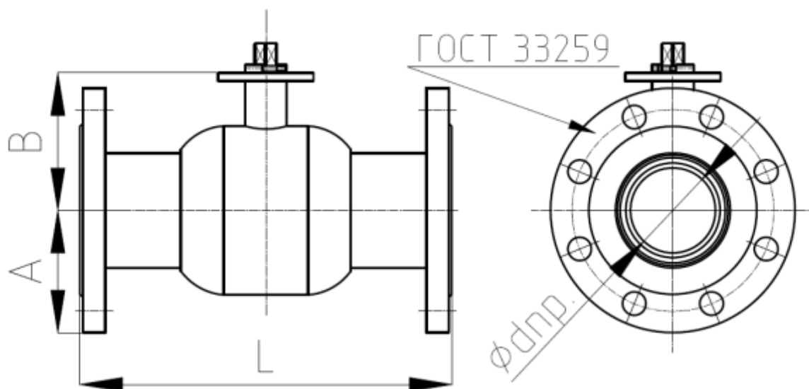
Габаритные и присоединительные размеры кранов шаровых типа RJIP в мм.
