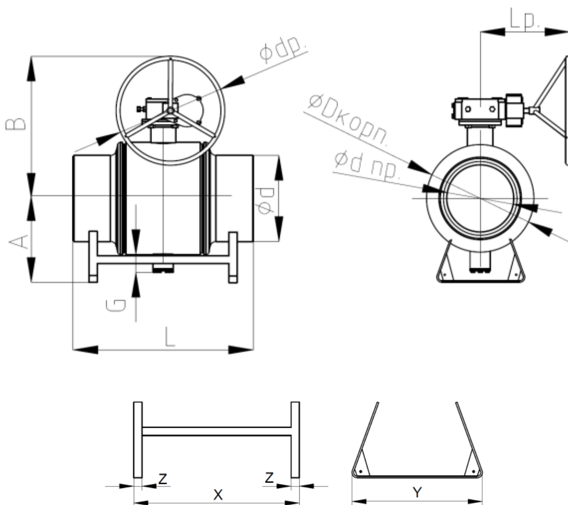
Габаритные и присоединительные размеры кранов шаровых типа RJIP в мм.
