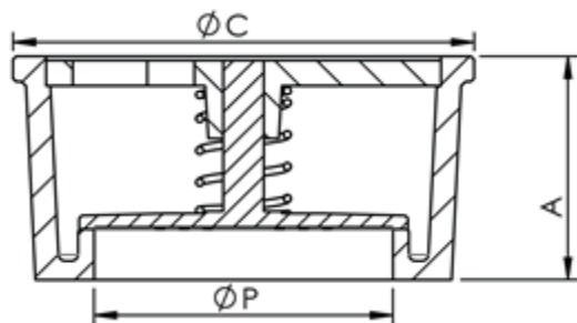
Габаритные и присоединительные размеры обратных затворов.
