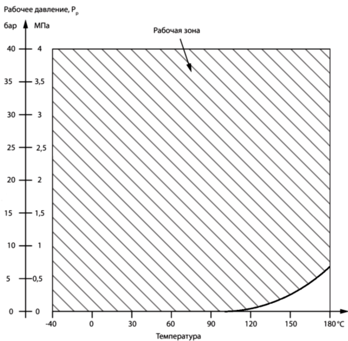
График Температура-Давление
