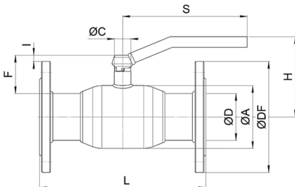
Габаритные и присоединительные размеры кранов шаровых типа RJIР, фланцевые.
