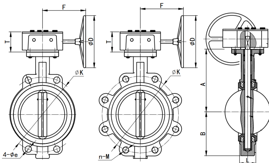
Габаритные и присоединительные размеры
