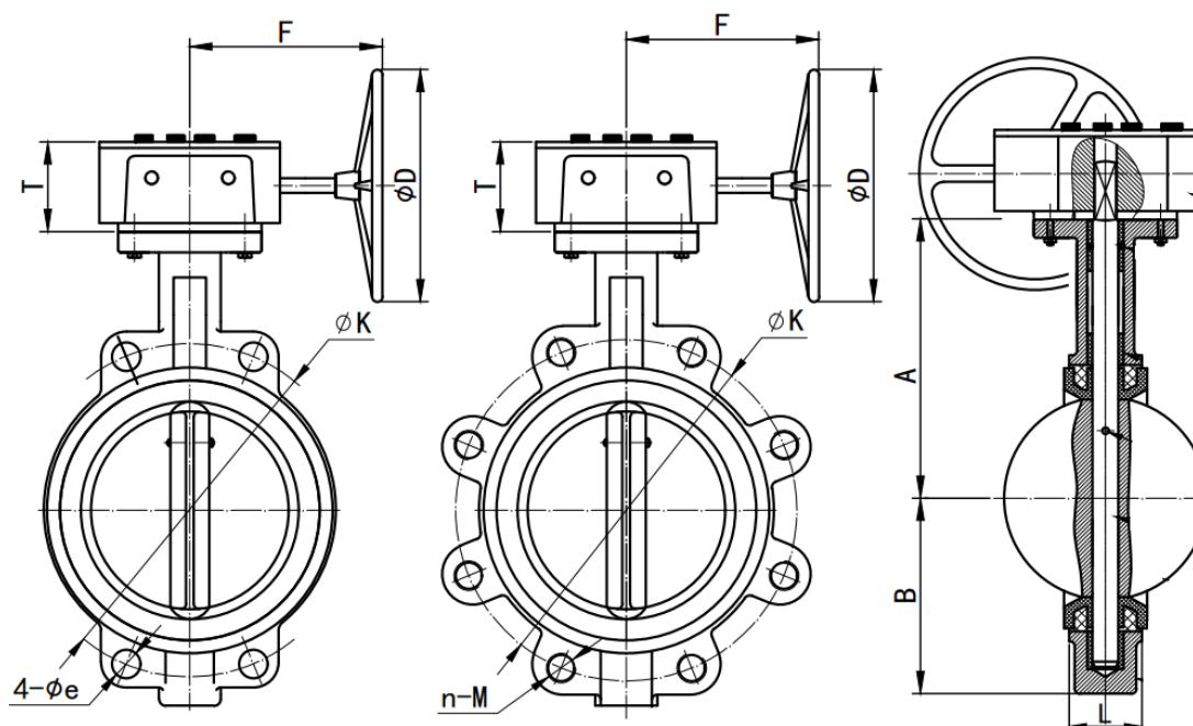
Габаритные и присоединительные размеры
