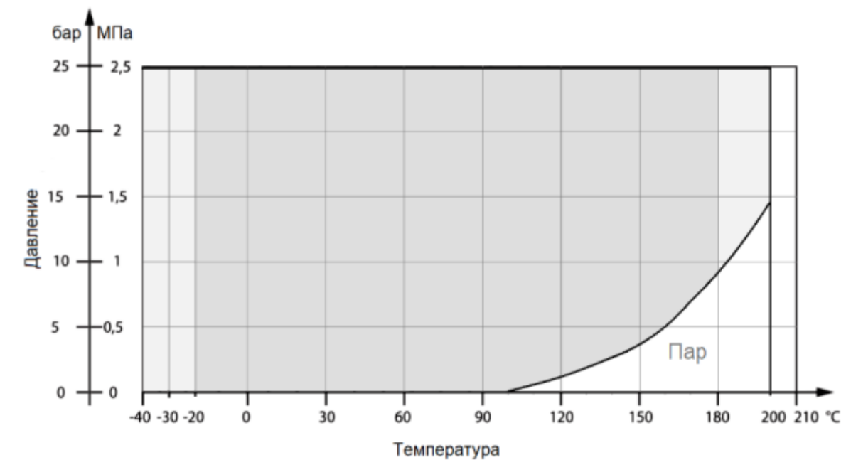
Диаграмма Температура-Давление
