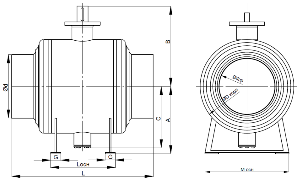
Габаритные и присоединительные размеры кранов шаровых типа RJIP, фланцевые.
