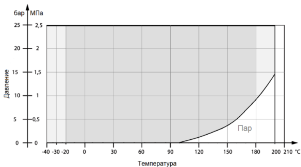
Диаграмма Температура-Давление
