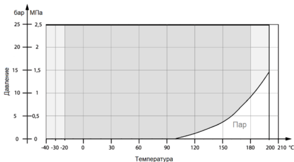
Диаграмма Температура-Давление
