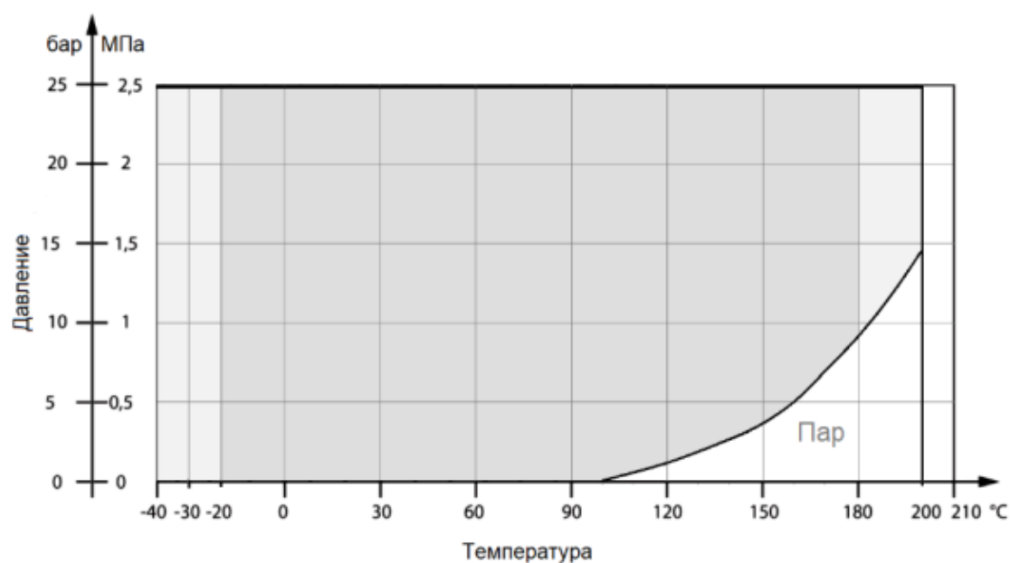
Диаграмма Температура-Давление
