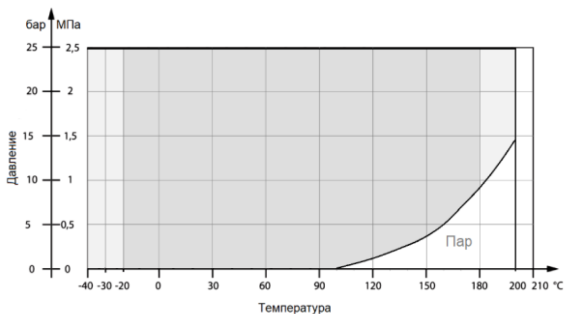
Диаграмма Температура-Давление
