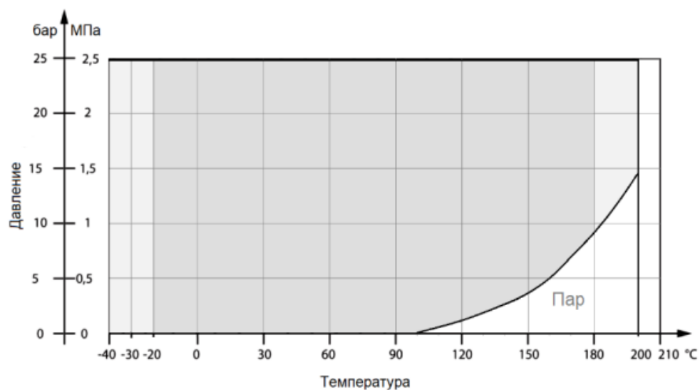
Диаграмма Температура-Давление
