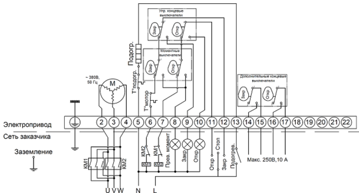
Рис. 3 - Электрические присоединения
