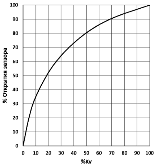
Диаграмма зависимости коэффициента пропускной способности K от степени открытия регулятора.
