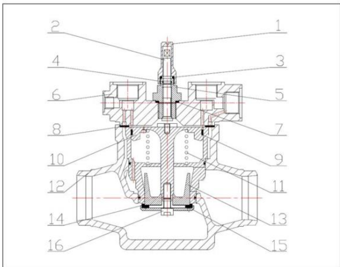
Рисунок 1. Конструкция
