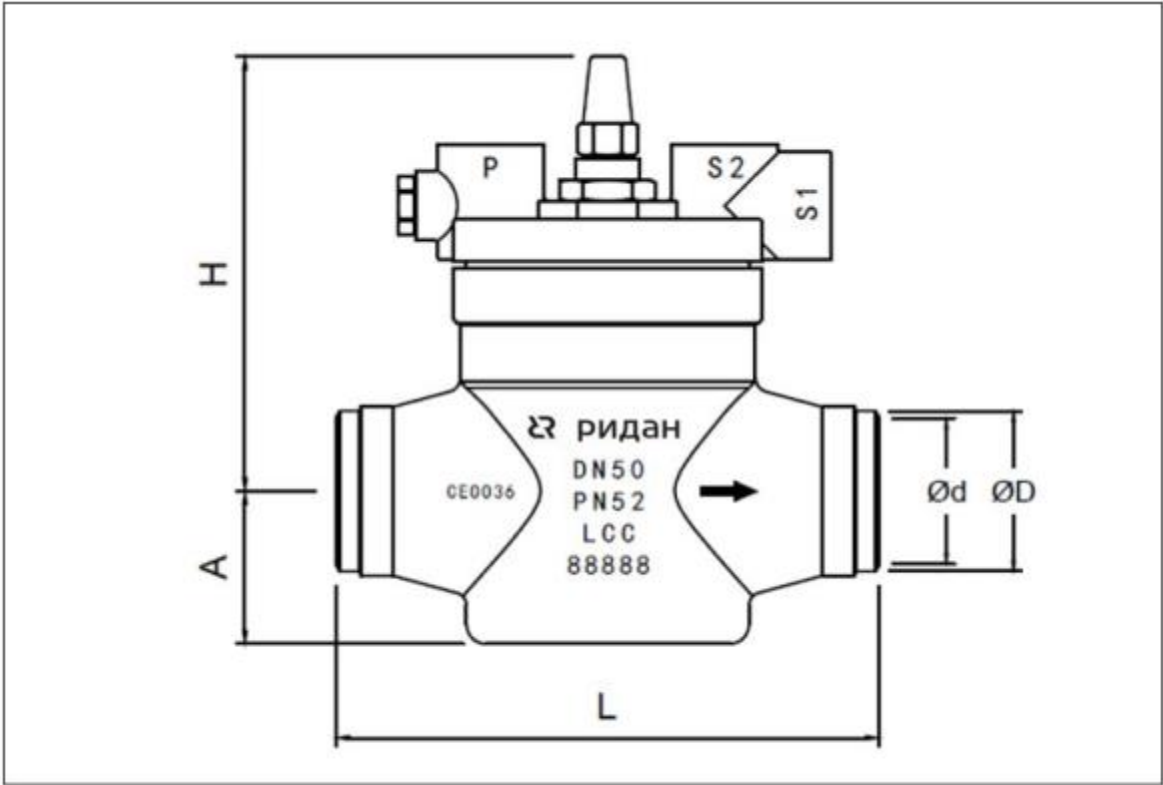
Рисунок 2. Размеры
