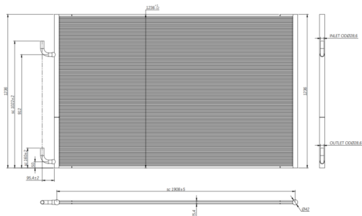
Габаритные размеры и изображение теплообменника микроканального модификации RC-1950.
