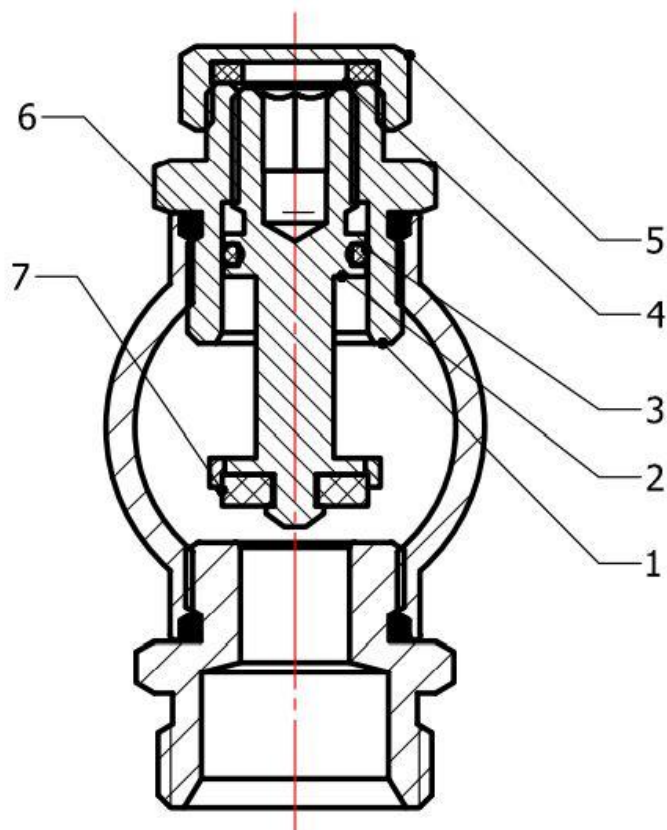
Рис. 1. Устройство подающей гребенки без ротаметров
