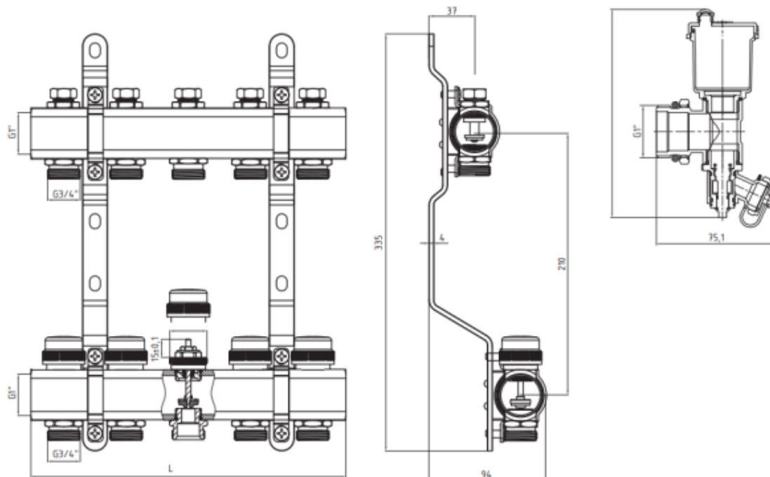
Рис. 1 - Коллекторы типа FHF (коллектор для подающего трубопровода - сверху, коллектор для обратного трубопровода - снизу)
